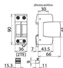
Dimensioni DG M TT 2P 275 FM
