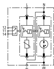
Schema di principio DG M TT 2P 275 FM
