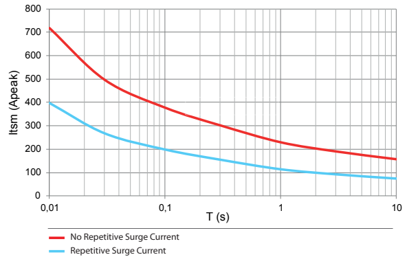
GN - 50 A Istantaneo
