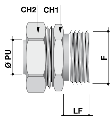
art. 6014 MASCHIO FISSO FIXED MALE
