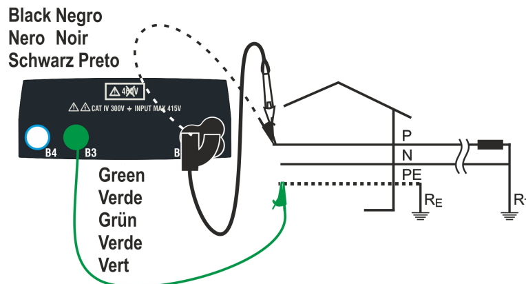
Fig. 29: Test 2 fili P-PE per sistemi monofase/bifase con cavi e puntale remoto
