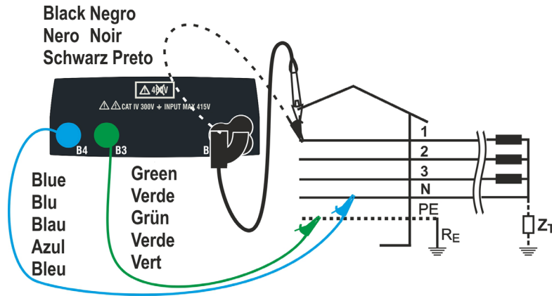
Fig. 27: Test P-PE per sistemi IT mediante cavi singoli e puntale remoto
