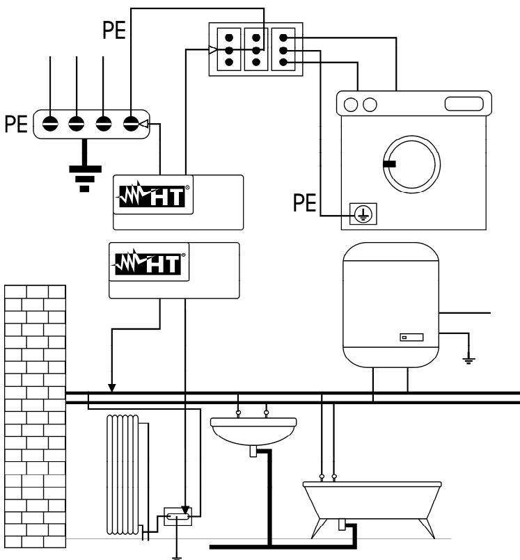
Fig. 35: Esempi di misure di continuità dei conduttori
