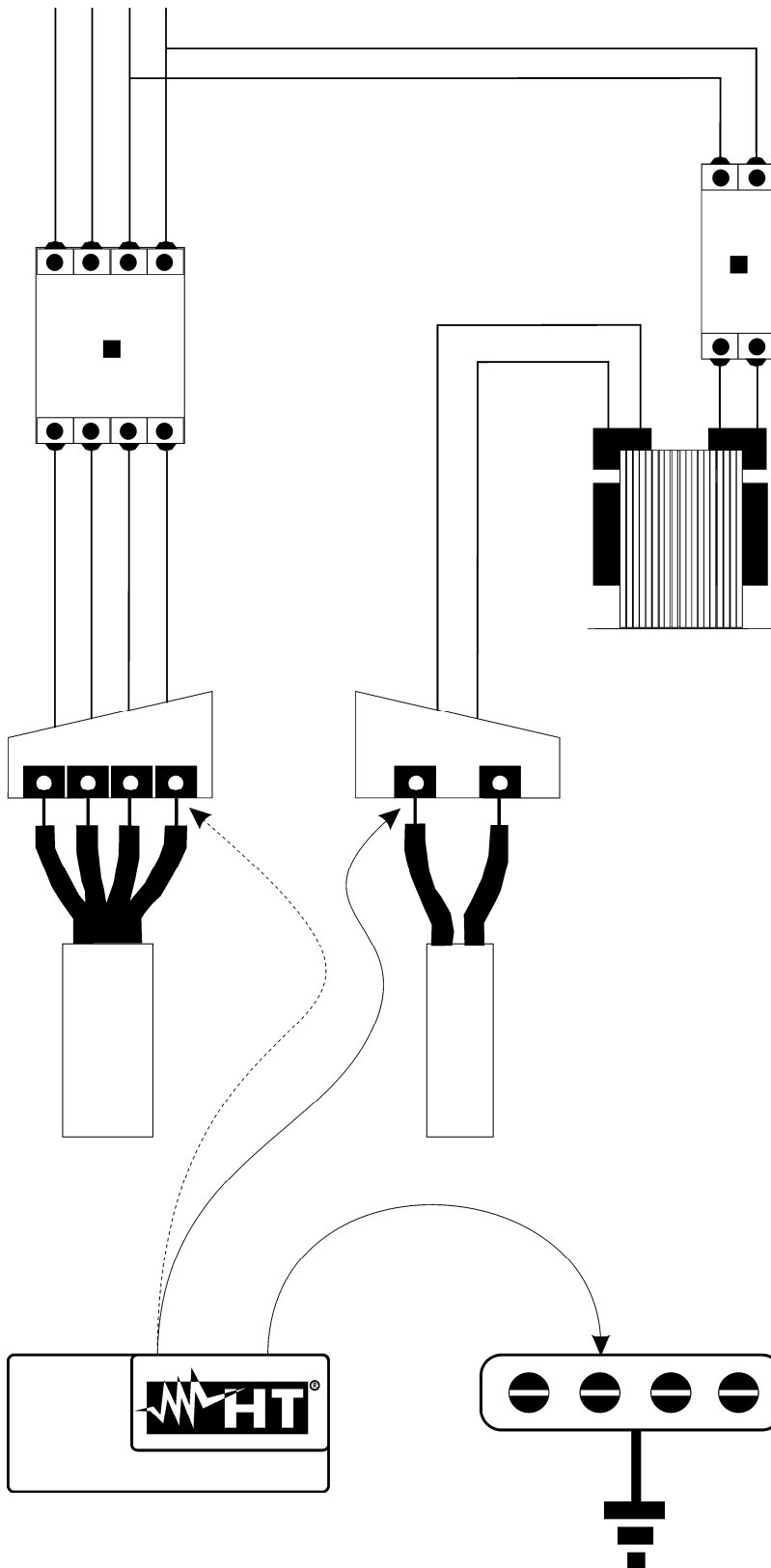
Fig. 36: Misure di separazione tra circuiti in un impianto
