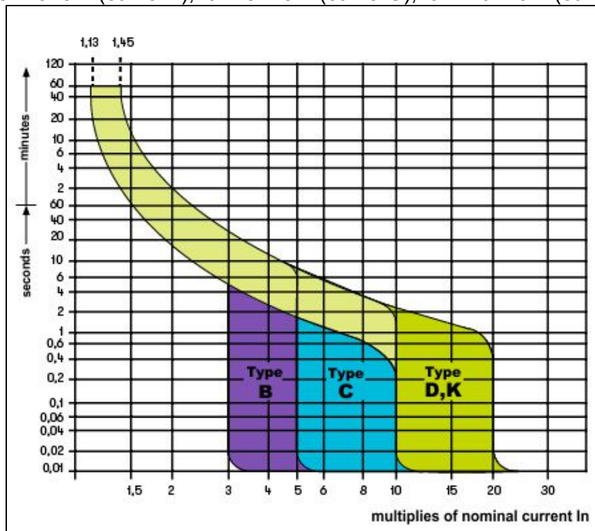
Fig. 37: Curve di intervento protezioni magnetotermiche (MCB)
