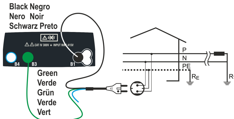
Fig. 28: Test P-PE 2 fili per sistemi 230V monofase/bifase con spina Shuko
