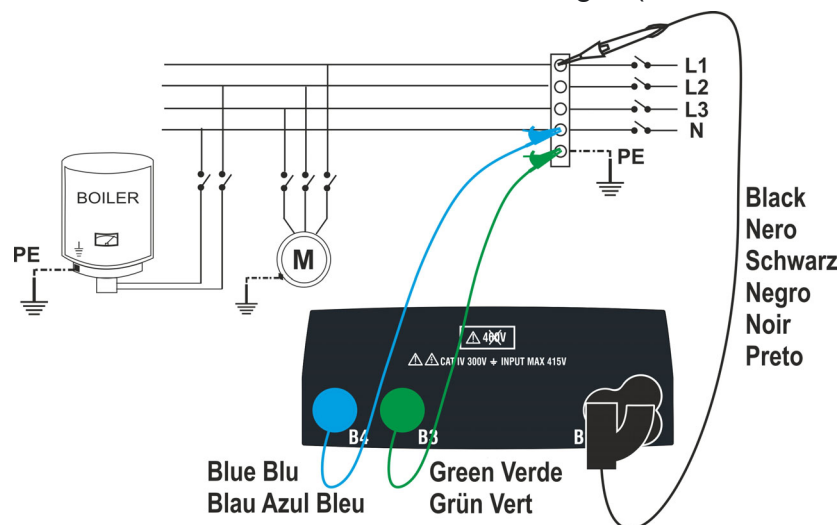
Fig. 11: Isolamento tra L-N-PE tramite cavi singoli (modi MAN e AUTO)
