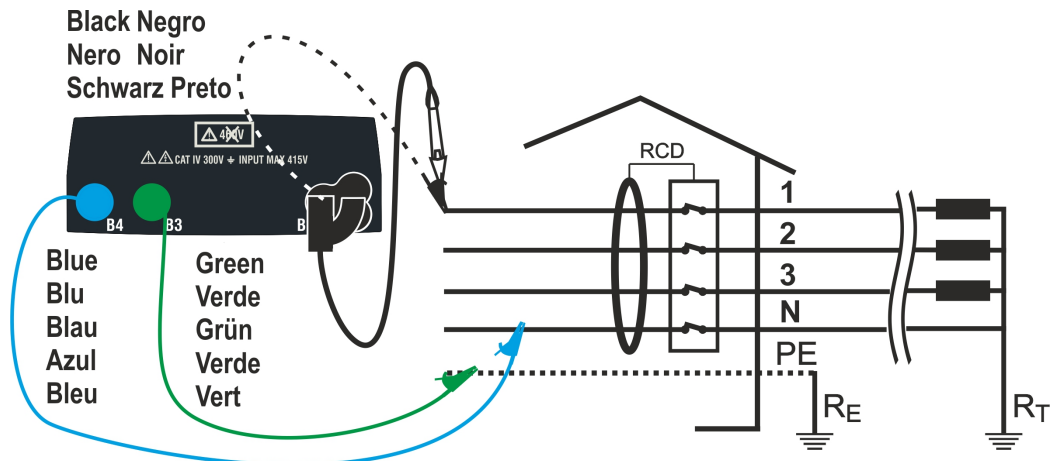
Fig. 19: Collegamento per sistema trifase 400V + N + PE tramite cavi singoli e puntale remoto
