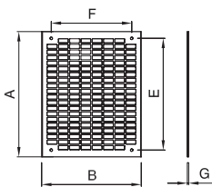
piastre forate in acciaio
