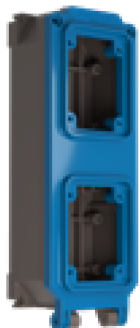
SERIE TAIS Contenitore da parete modulare con sistema TAIS per 2 frutti safety performance IP66/IP67/IP68/IP69
