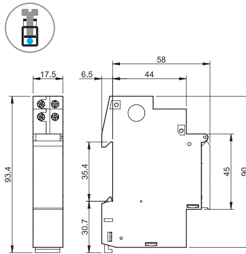
Tipo 12.11 Morsetti a vite
