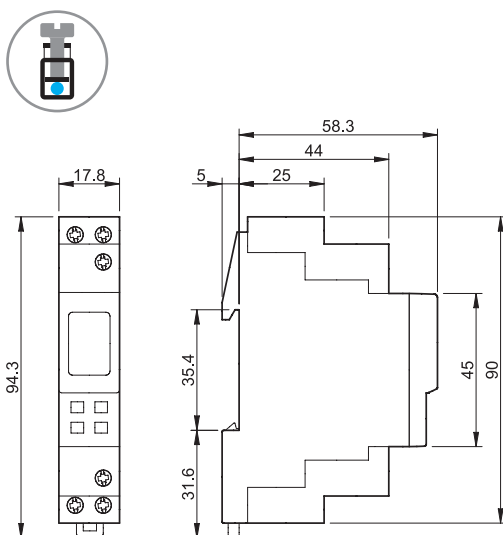
Tipo 12.71 Morsetti a vite
