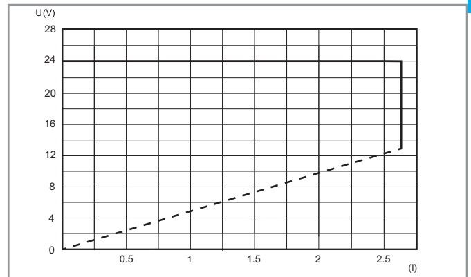
FB78-2 Tensione di uscita in funzione della corrente di uscita (78.60)
