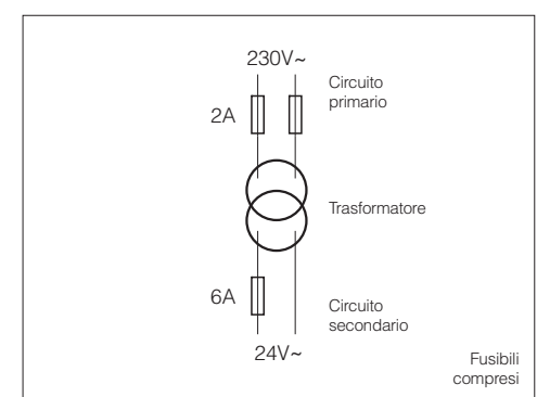
Protezioni previste per la versione LARGE con trasformatore.
