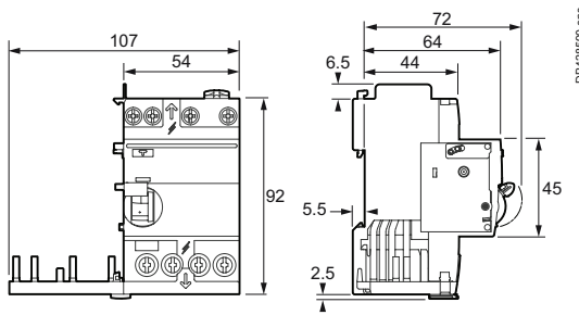
Vigi iCG40 "Gruppo di partenze" 3P+N
