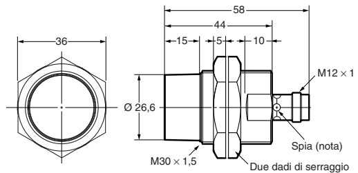
E2A-M30KN20-M1-□□/E2A-S30KN20-M1-□
